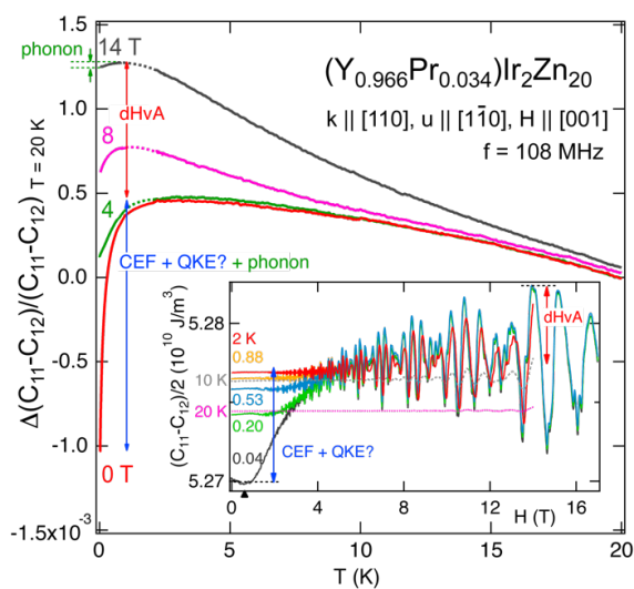
図 3. Y_{0.966}Pr_{0.034}Ir_2Zn_{20} の横波弾性率 (C_{11}-C_{12})/2 の温度変化と磁場変化に現れる量子振動（内挿図）。縦軸は物質の「硬さ」に対応するため、温度を下げると（グラフの左側に行くほど）、徐々に硬くなっていた物質が急激に「柔らかく」なっていることがわかる。
